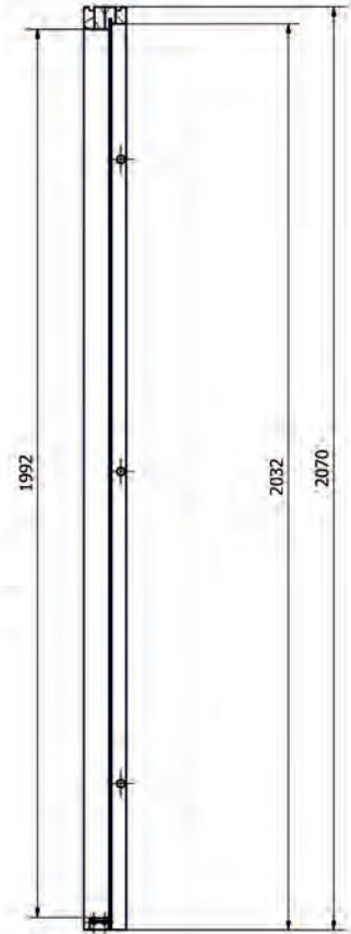
B-B (1 : 8)
