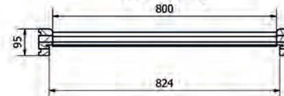
A-A (1 : 8)
